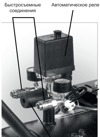
Рис. 4 Регулятор давления
